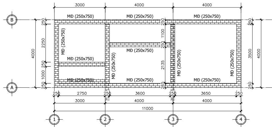
MẶT BẰNG MÓNG ĐÁ CHÈ
