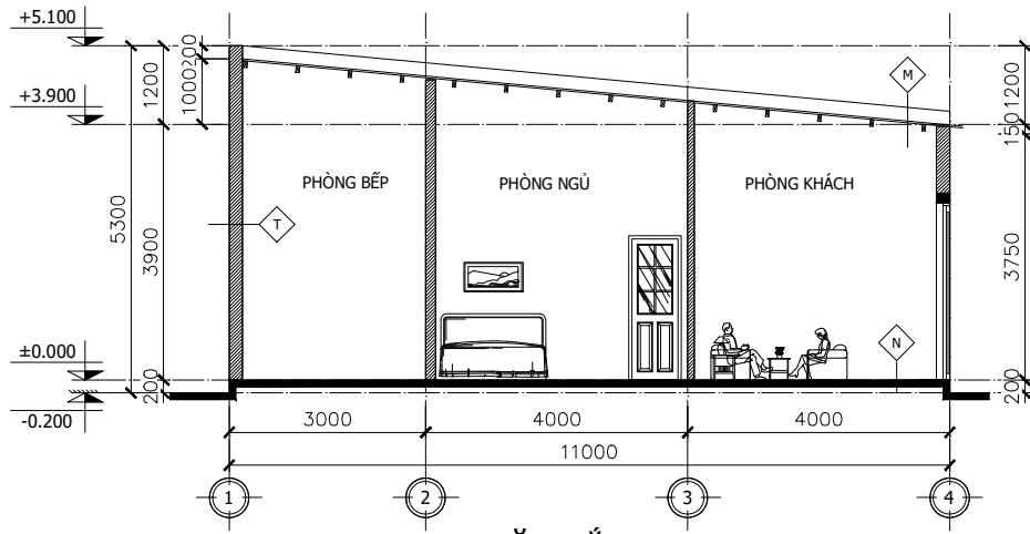
MẶT CẮT A-A TL: 1/100
