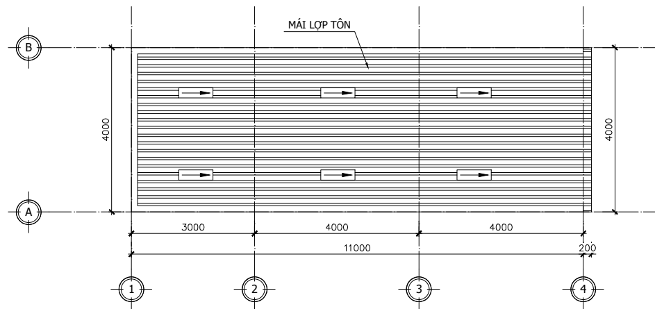
MẶT BẰNG MÁI
