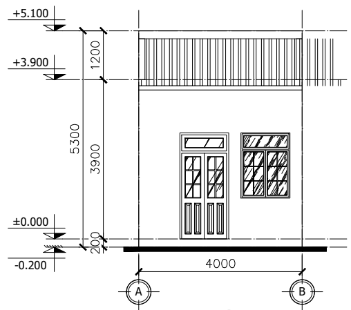
MẶT ĐỨNG A-B TL: 1/100
