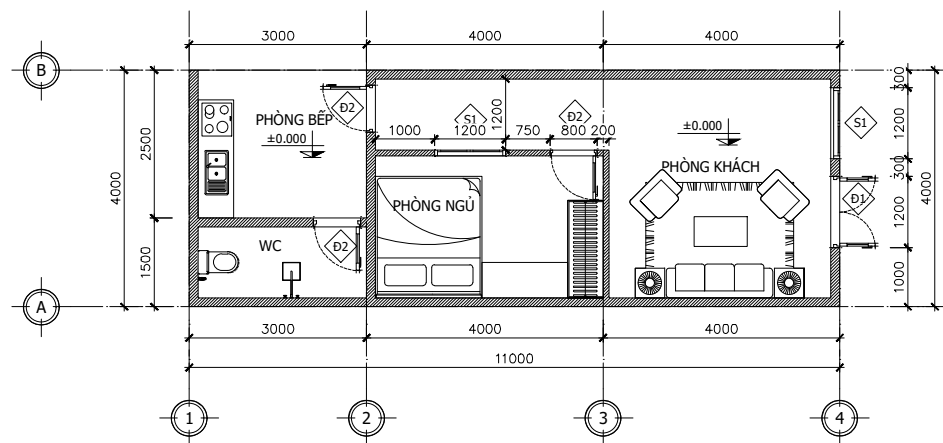
MẶT BẰNG TẦNG 1
