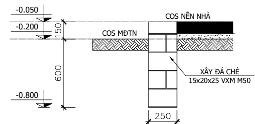
MÓNG ĐÁ CHÈ MĐ
