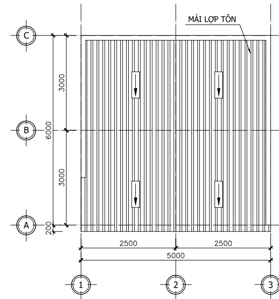
MẶT BẰNG MÁI
