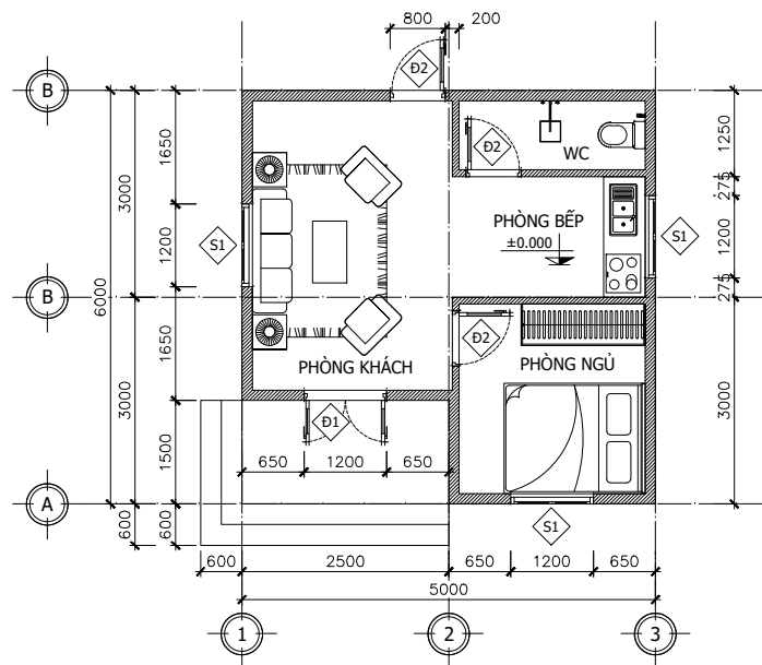
MẶT BẰNG TẦNG 1
