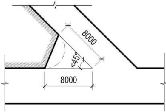
a) Kích thước vạt góc tại góc cắt giao nhau với lộ giới nhỏ hơn 45^0
