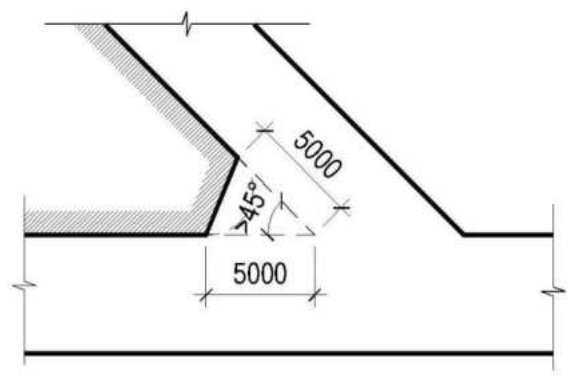
b) Kích thước vạt góc tại góc cắt giao nhau với lộ giới lớn hơn hoặc bằng 45^0
