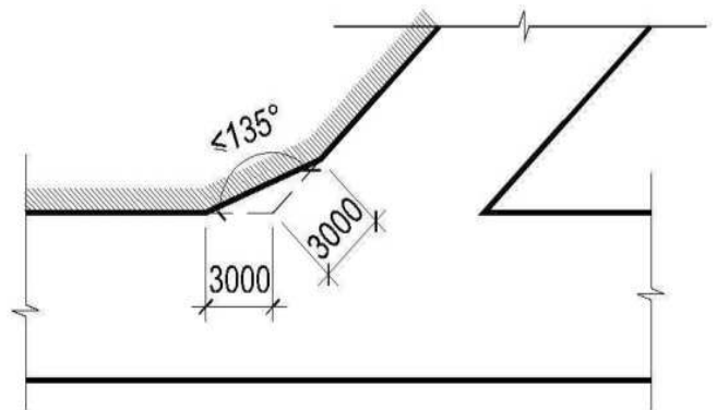
d) Kích thước vạt góc tại góc cắt giao nhau với lộ giới nhỏ hơn hoặc bằng 135^0
