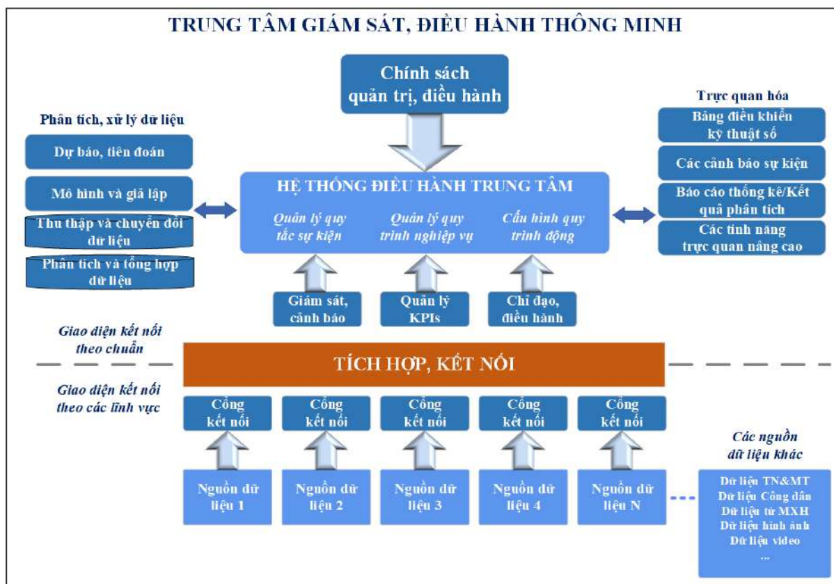
Hình 9: Mô hình tổng thể trung tâm giám sát, điều hành ĐTTM
